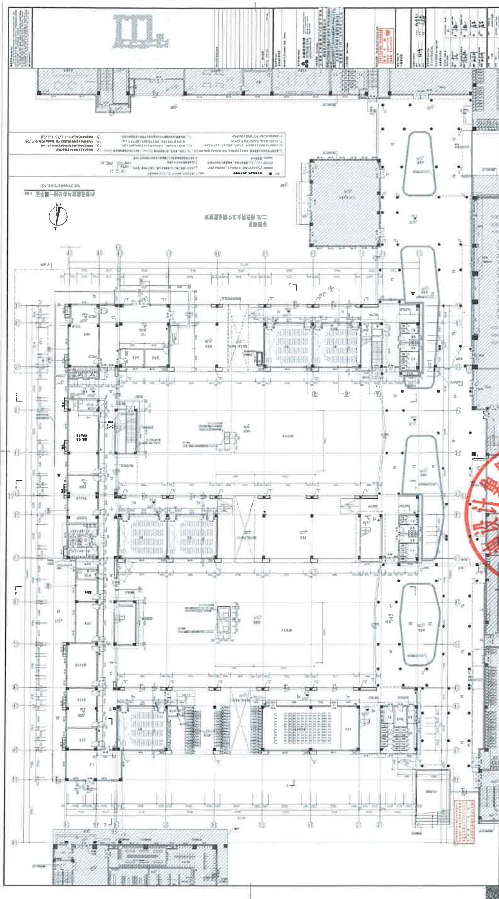
图纸 A-01A-0100_一层平面图(第4版)
