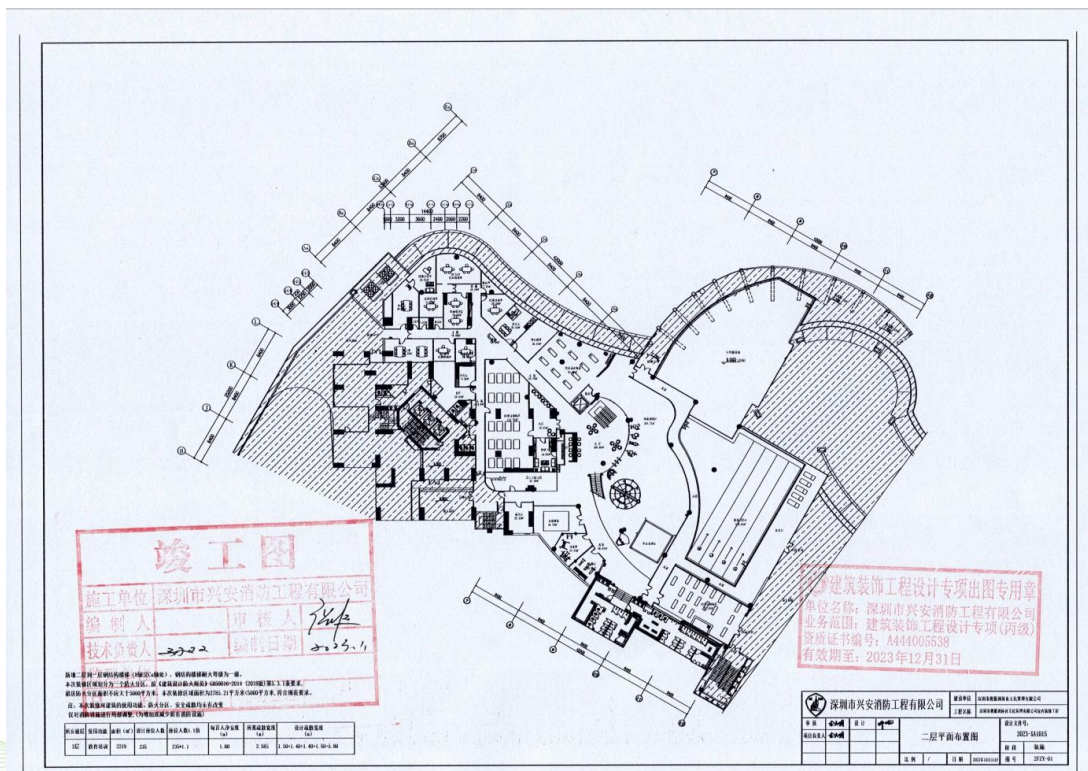
自运营室内文体场馆平面图 (二层)
