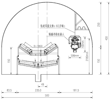
图 7.4-1 隧道主洞建筑限界（单位：cm）
