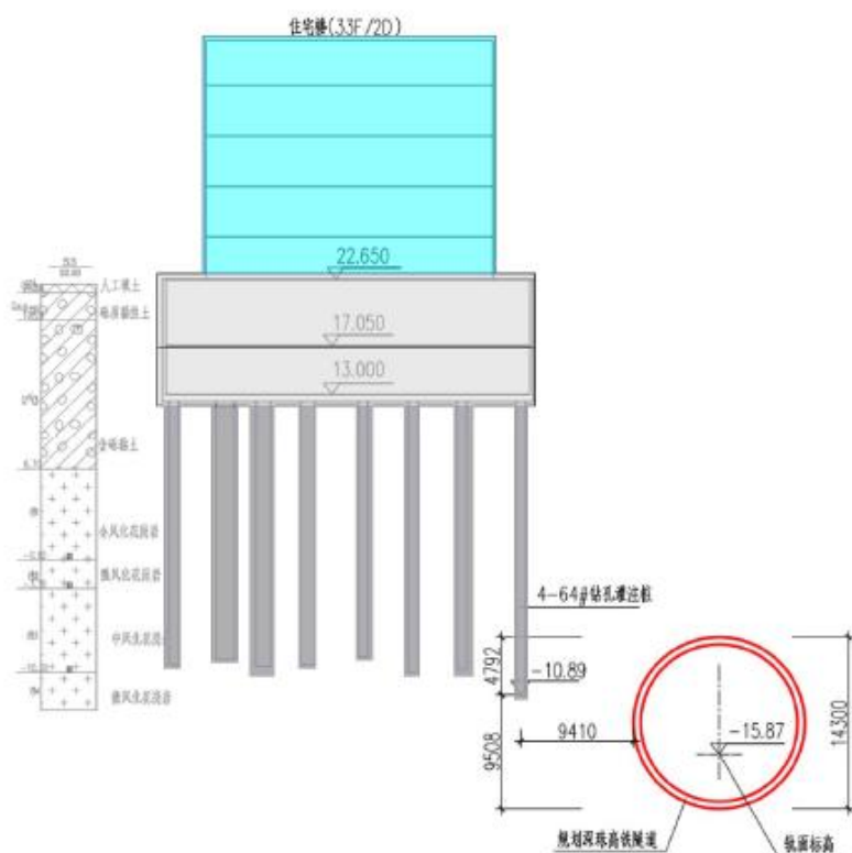
图 1.4.4 南山建工村建筑物与深珠高铁横剖面关系图（二）
