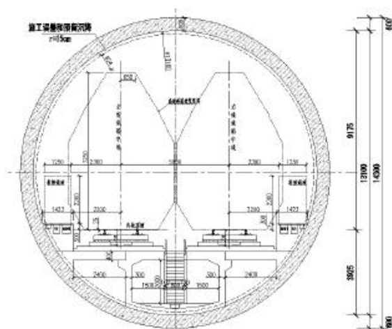
图 1.2.1 单洞双线铁路盾构隧道横断面
