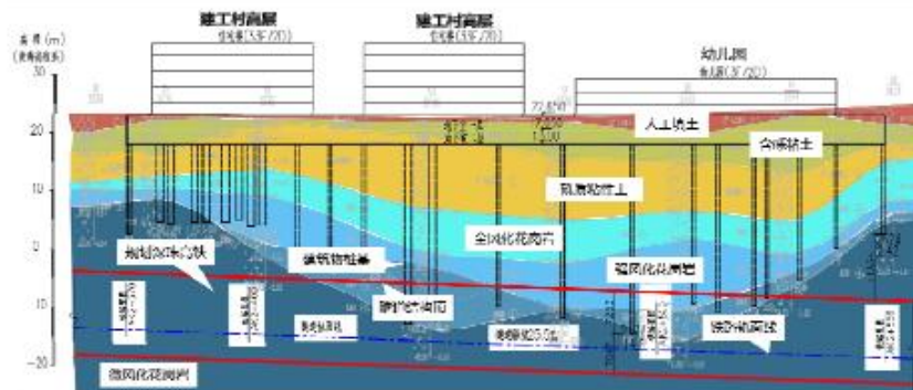
图 1.4.2 南山建工村建筑物与深珠高铁纵剖面关系图
