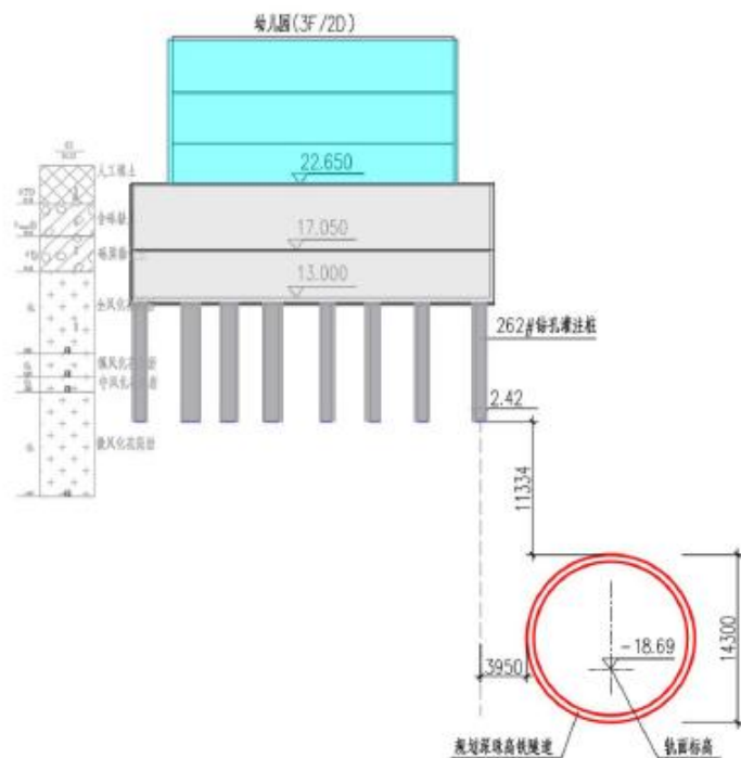
图 1.4.3 南山建工村建筑物与深珠高铁横剖面关系图（一）
