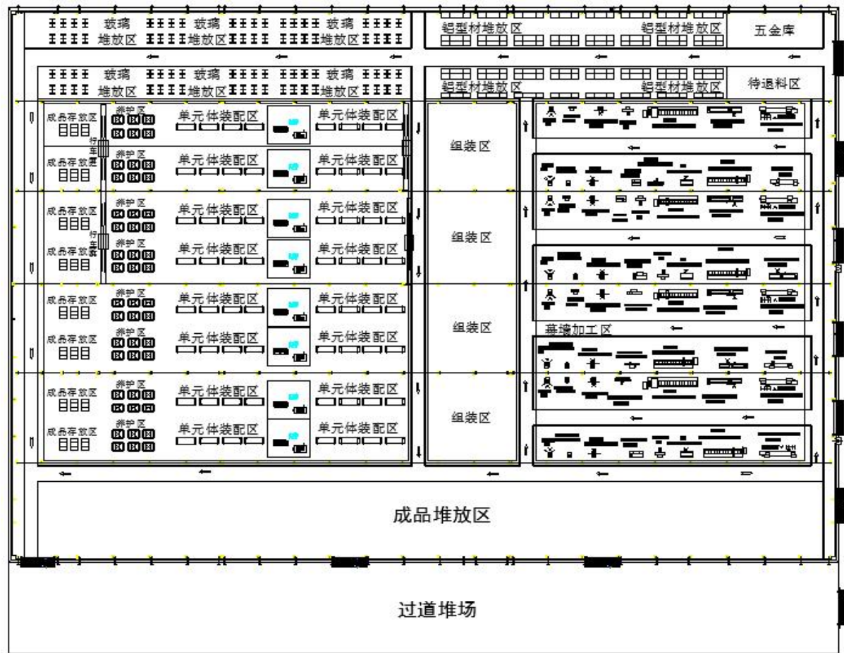
厂房加工区域布置图
