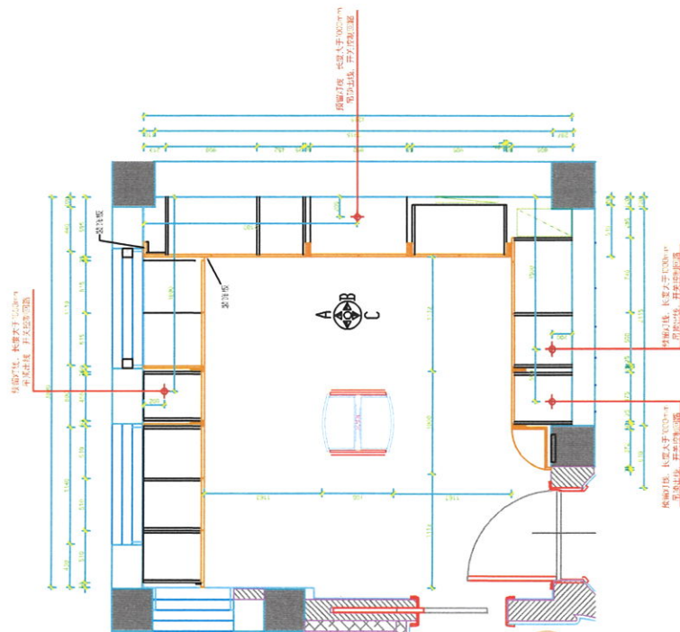
平面图
