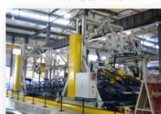
上/下导轨总成
