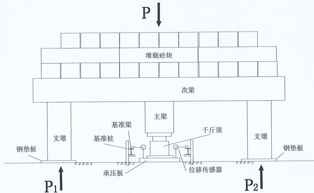
图 1 加载装置示意图
