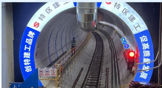
▲ 深圳市城市轨道交通16号线二期工程五工区：位于龙岗区园山街道，项目包含一站两区间，即：园山站-阿波罗站-阿波罗南区间和阿波罗南站-园山站区间
