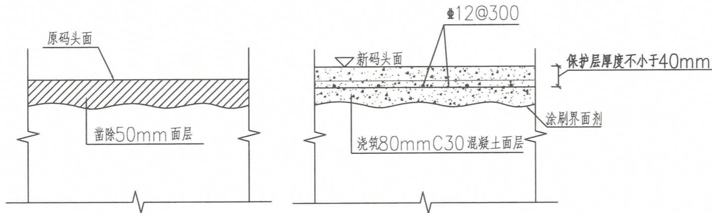
面层修复示意图
