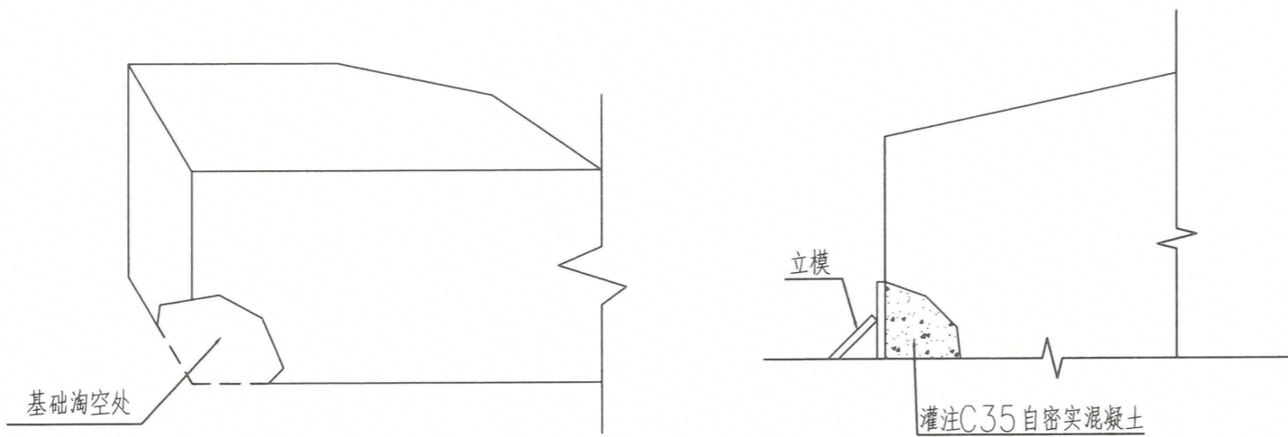
基础修复示意图
