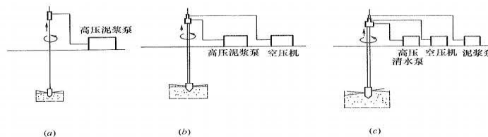
图 10-2 喷射注浆法施工工艺流程 (a) 单管法；(b) 二重管法；(c) 三重管法
