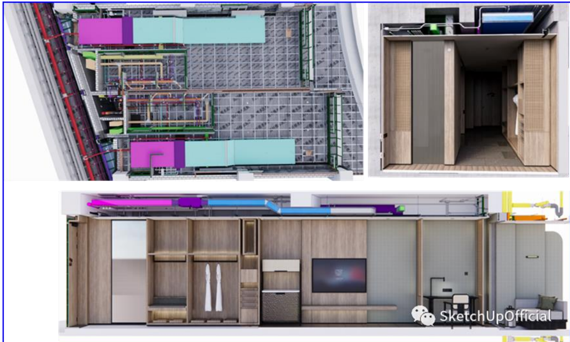
截图 1 建筑结构与精装 BIM、机电 BIM 进行碰撞检查
