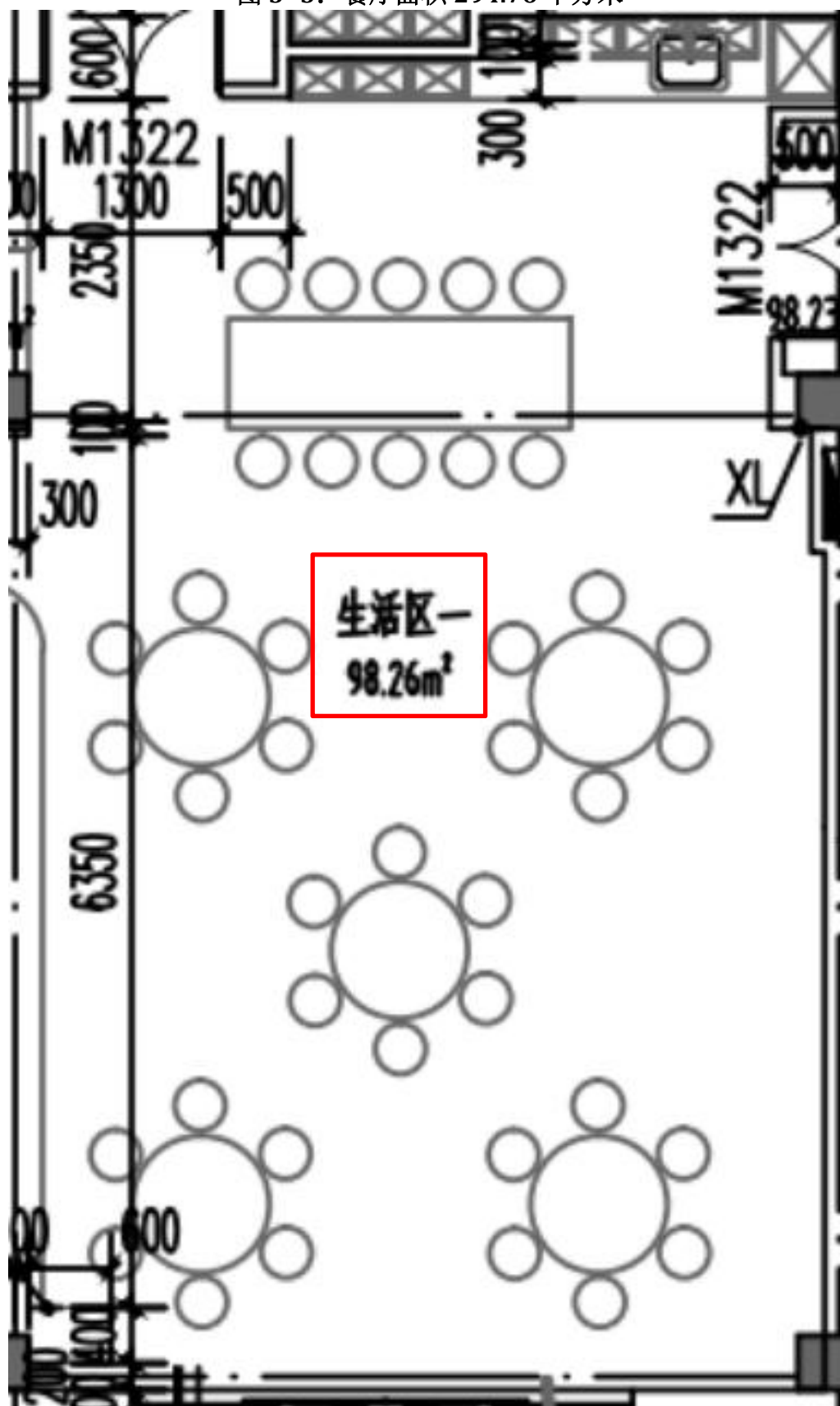
图 3~5：餐厅面积 294.76 平方米
