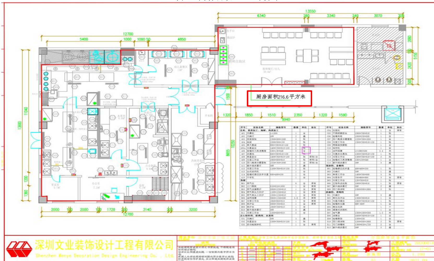
图 2: 厨房面积 216.6 平方米
