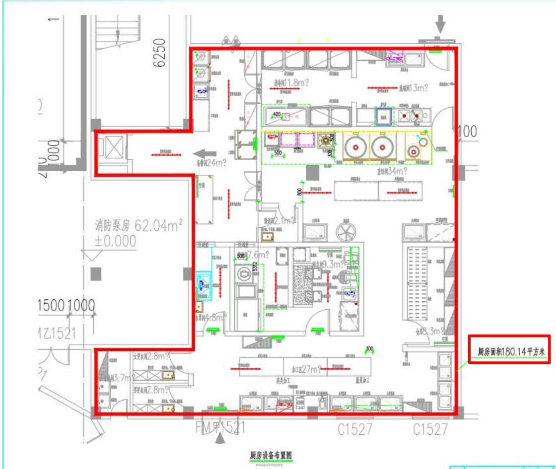
图 2：厨房面积 180.14 平方米
