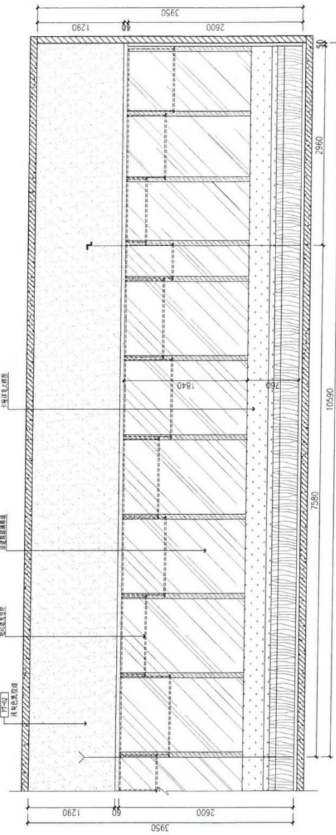
餐厅立面图 SCALE: 1:30
