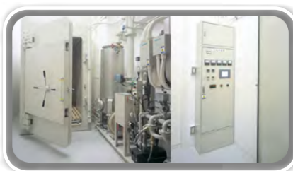
文物熏蒸室 2
