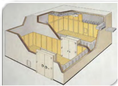
熊平恒温恒湿文物库示意图
