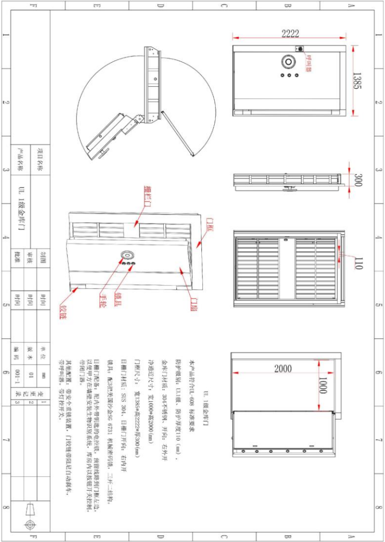
附件 2：金库门立面图
