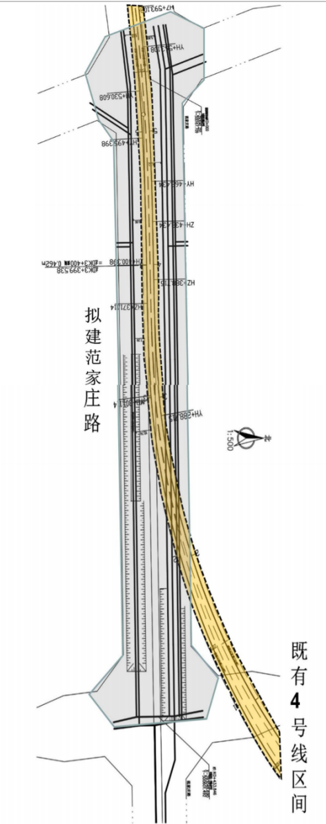
图 1.1-2 新建工程与地铁平面总平面关系图
