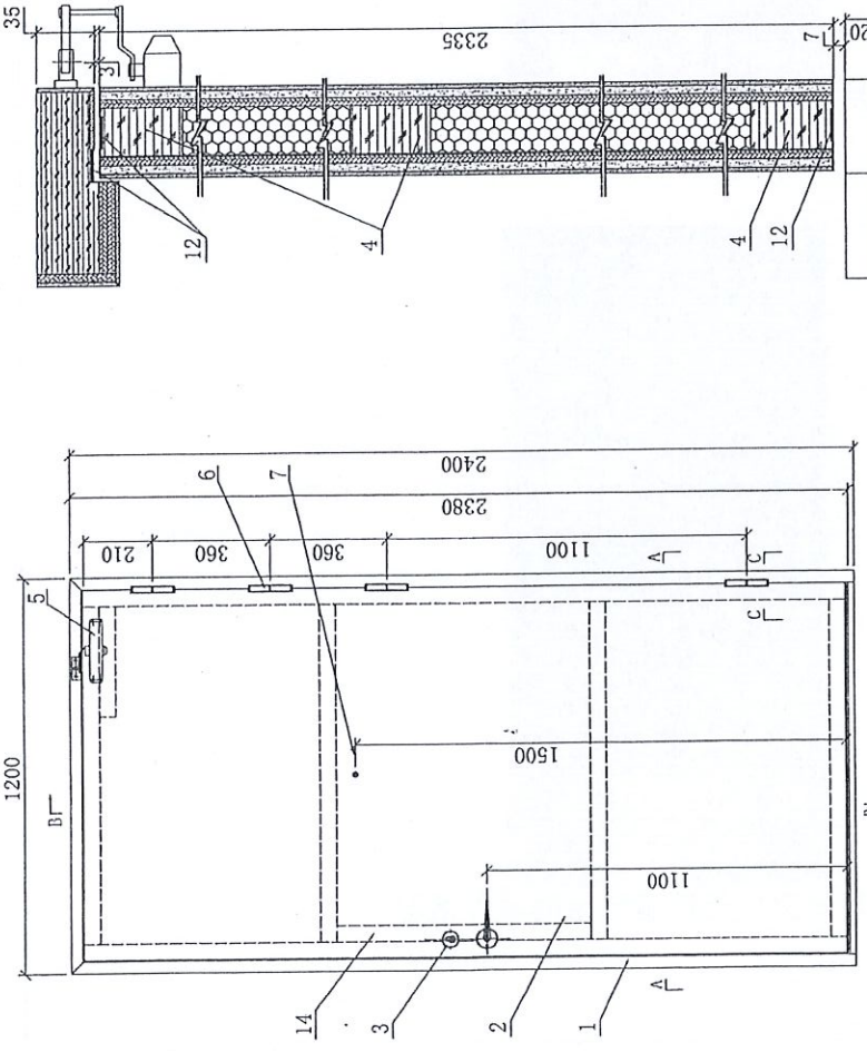
立面图
