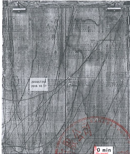
照片 1 耐火性能试验前试件情况
