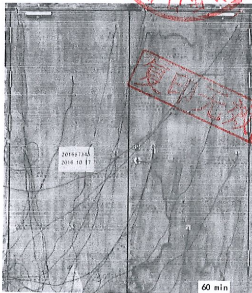
照片 2 耐火性能试验结束时试件情况
