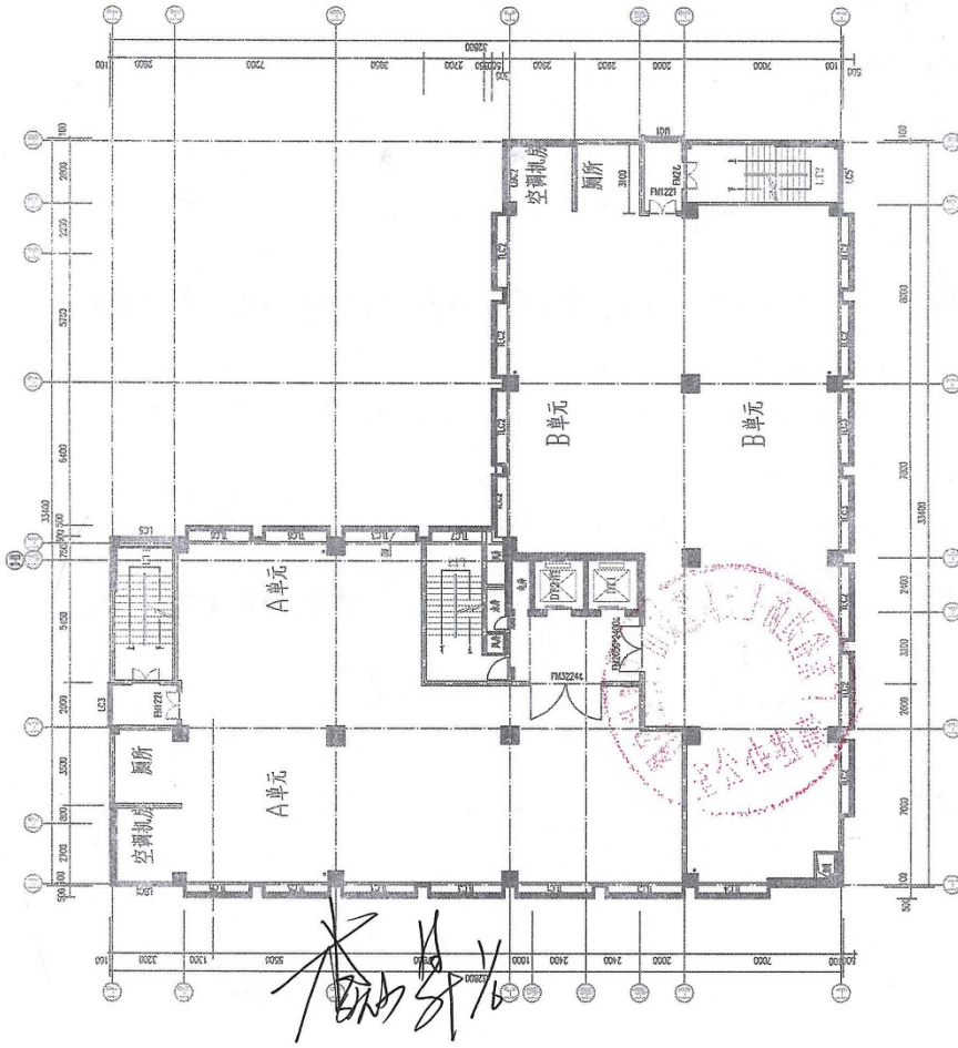
11楼平面图
