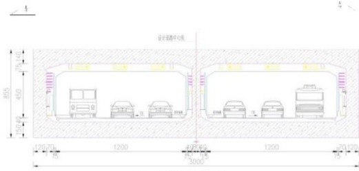
图 1-5 隧道暗埋段断面图
