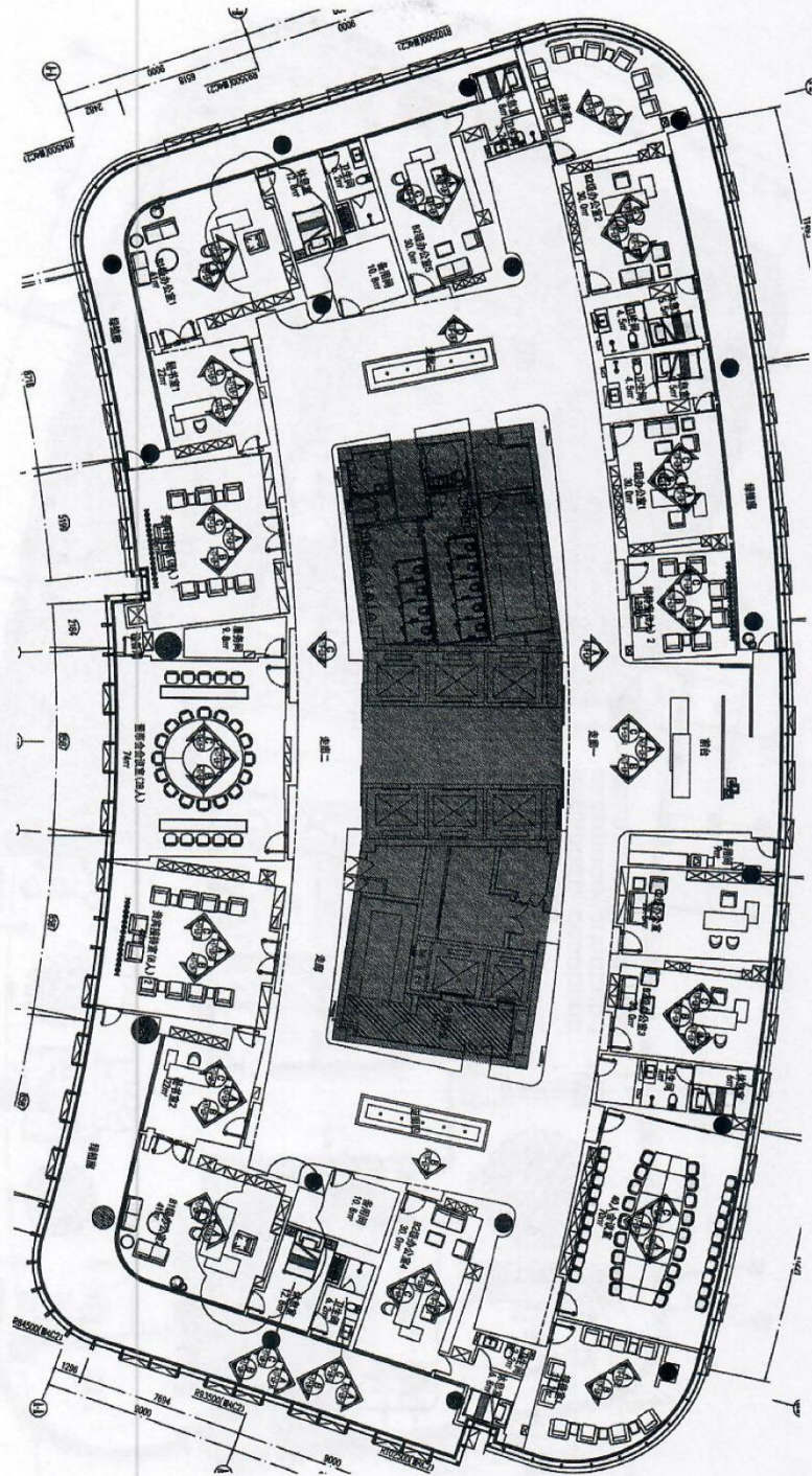
A座17层平面图
