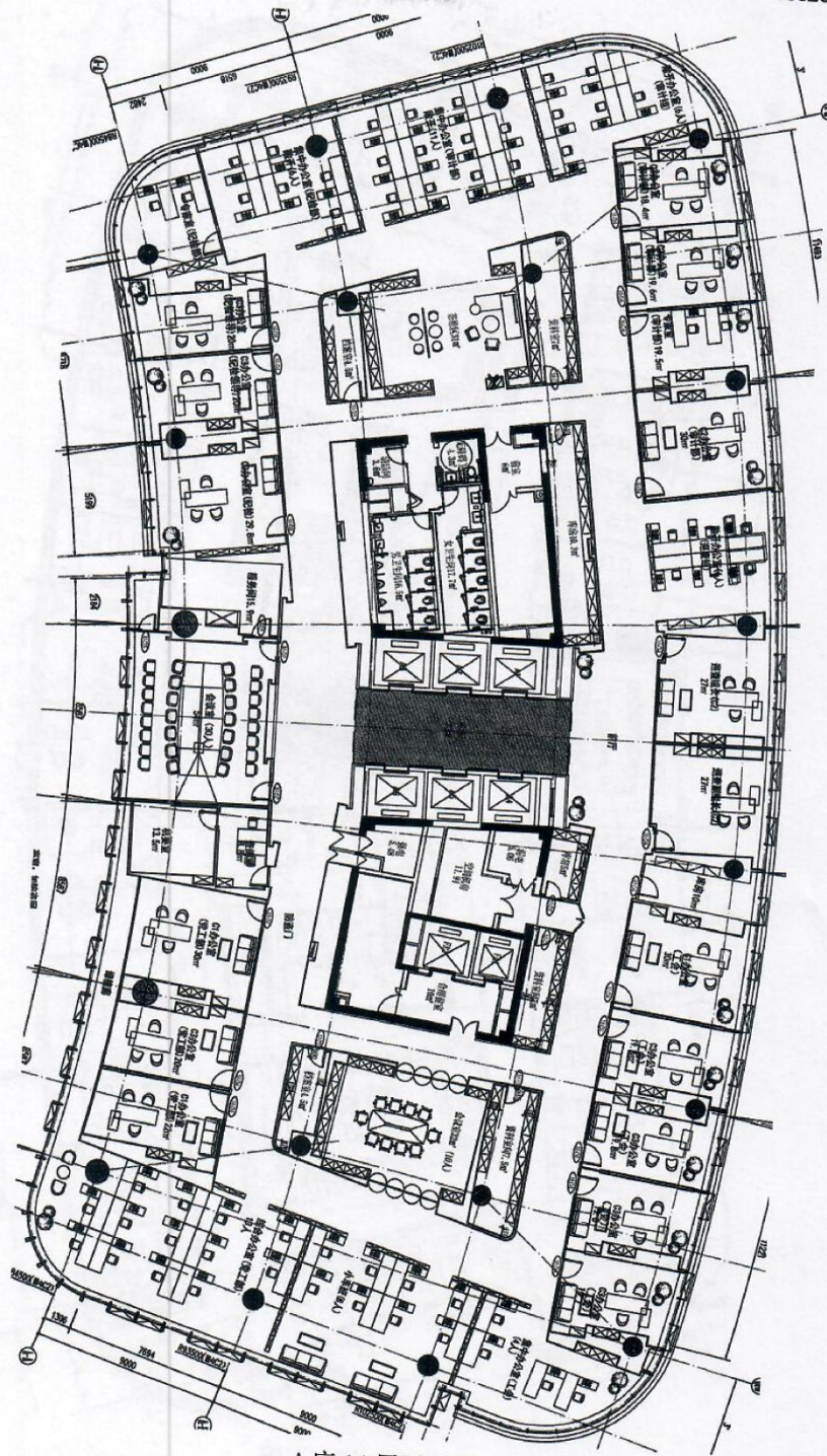
A座14层平面图
