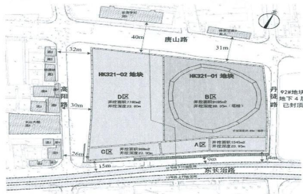
图1 基坑总平面布置
