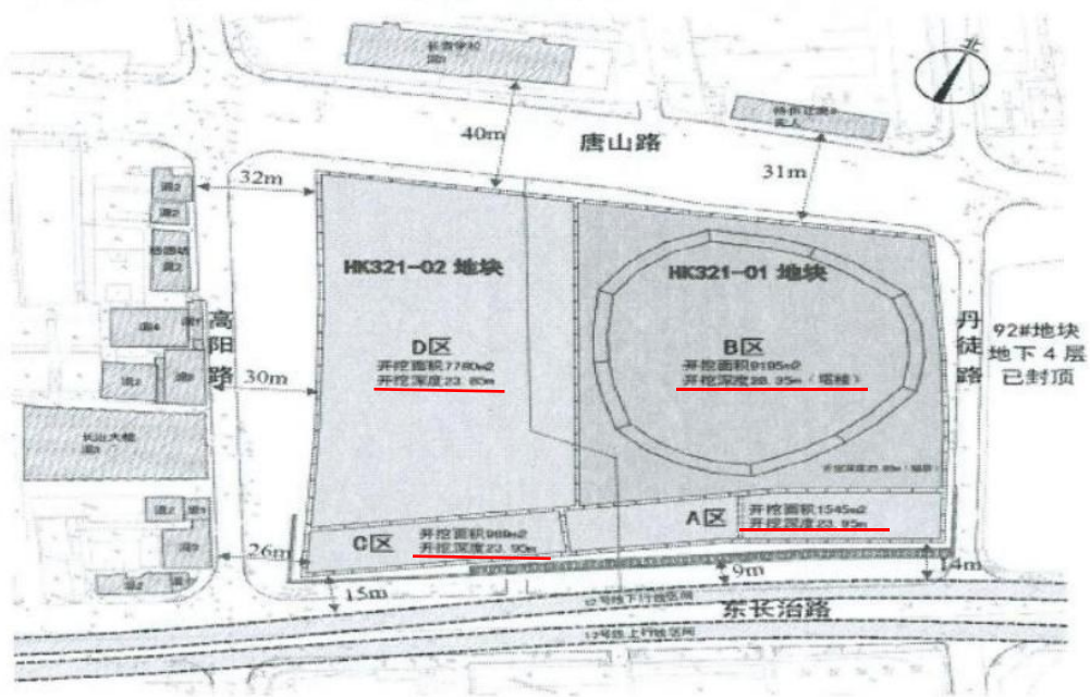
图1 基坑总平面布置
