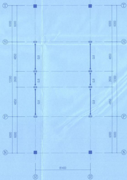
六层中庭屋盖 夹层结构平面图(二) 1:150
