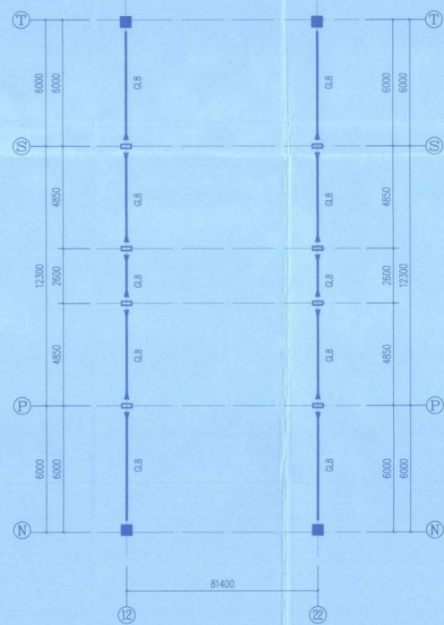
六层中庭屋盖 夹层结构平面图(一) 1:150
