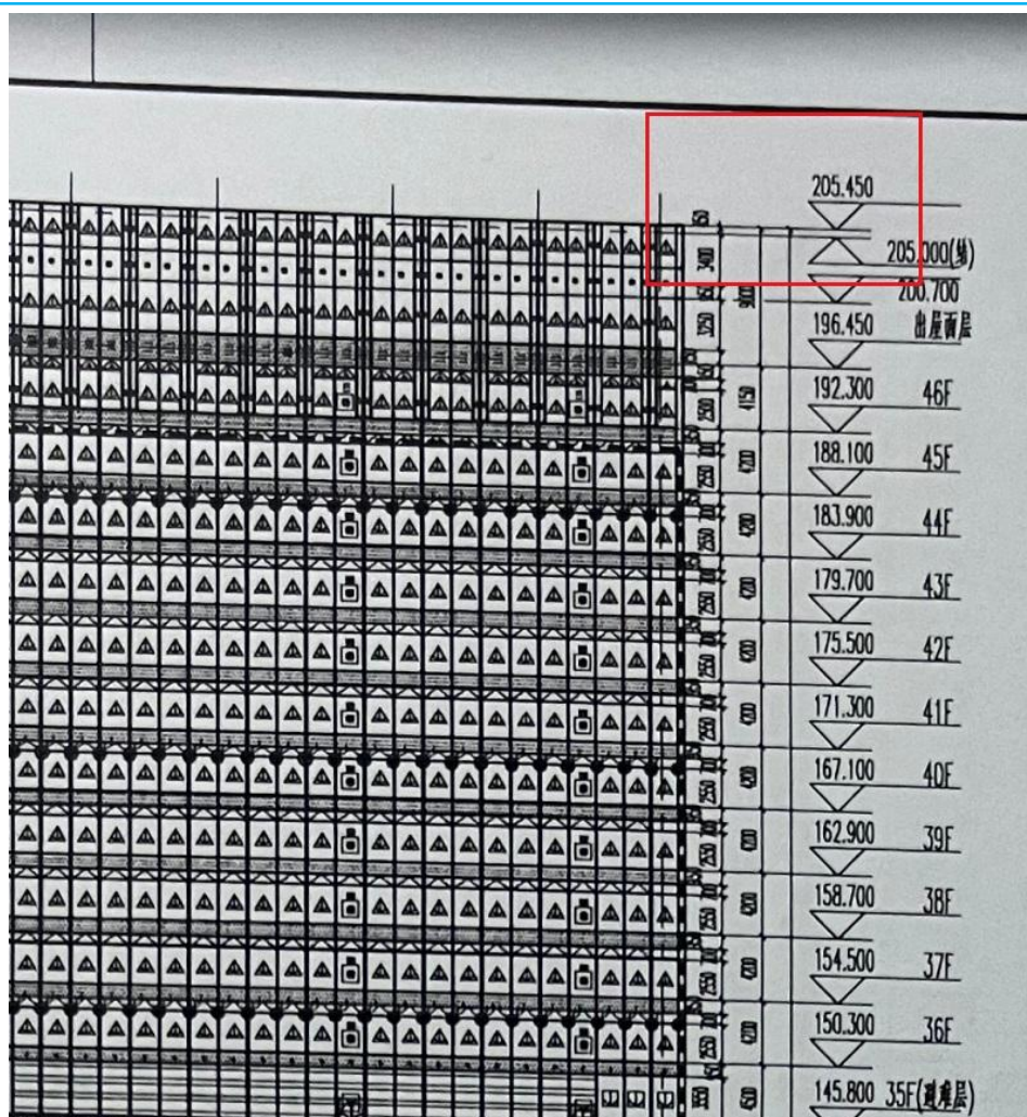
局部大样图
