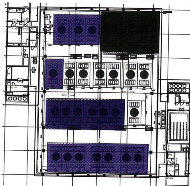
冷却塔层平面示意图（紫色阴影区域冷却塔非本次招标实施范围、冷却塔由发包人提供）
