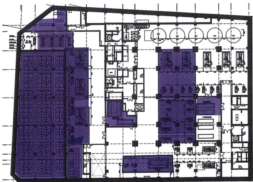
6号供冷站-3层平面示意图 (紫色阴影区域设备非本次招标实施范围, 制冷主机由发包人提供)
