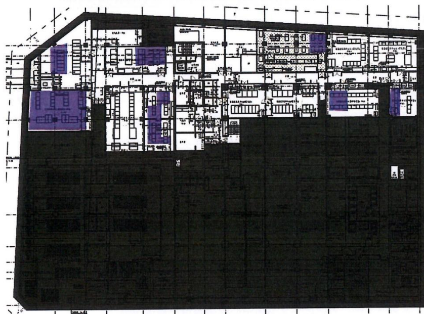
6号供冷站-2层平面示意图 (黑色阴影区域非冷站范围、紫色阴影区域电气设备非本次招标实施范围)
