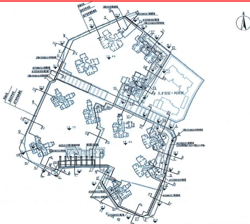
图 1-1 支护结构平面布置图
