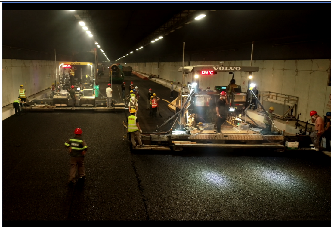
桂庙路快速化改造工程 3D 技术应用于隧道内路面项目
