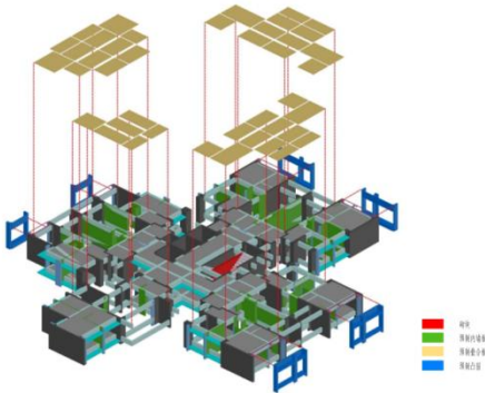
图 1.3-1 1 栋二单元标准层预制构件三维拆分图
