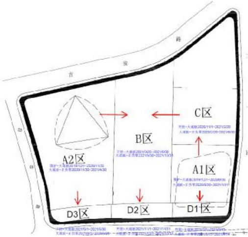
基坑分块示意图
