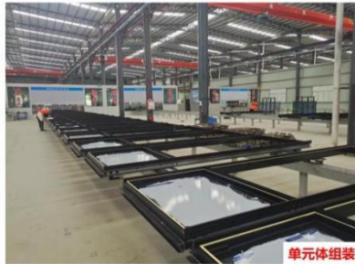
单元体组装
