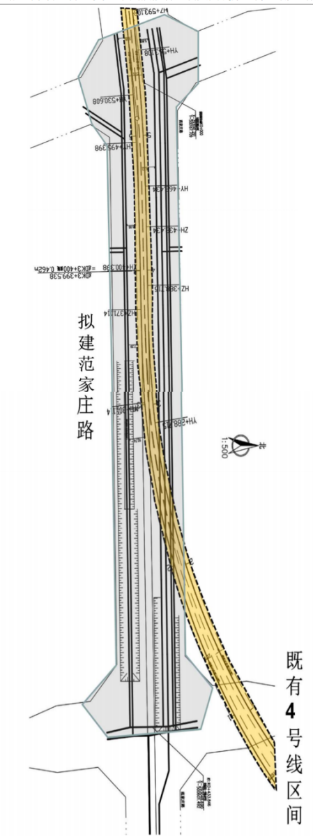
图 1.1-2 新建工程与地铁平面总平面关系图
