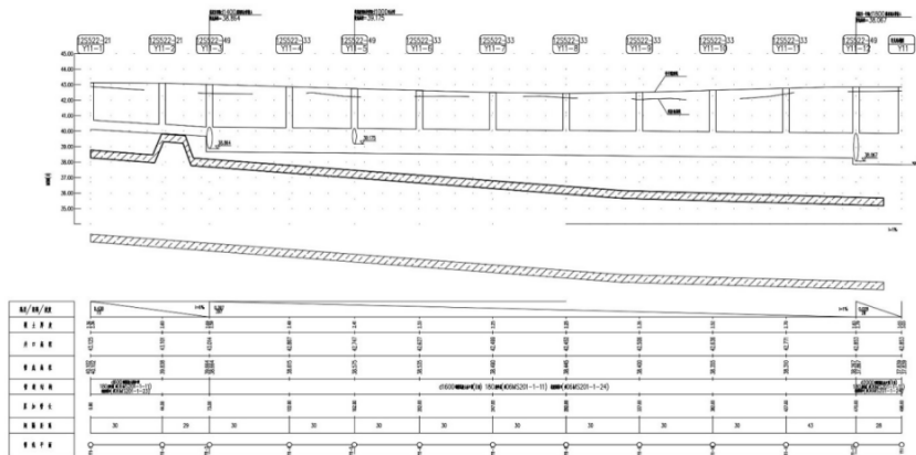
图 1.1-4 新建管线支线与地铁纵断面关系图
