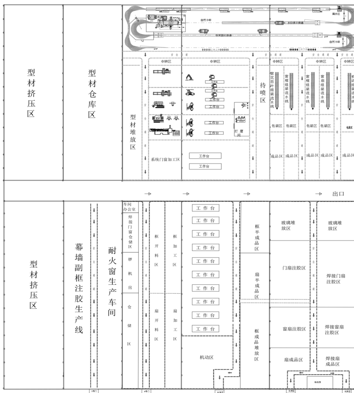
加工内部平面布置图
