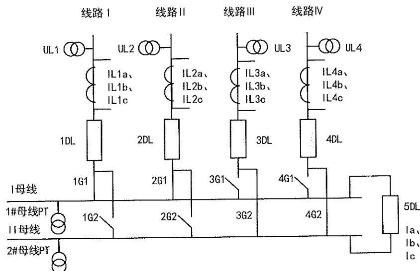
图 3 分段（母联）备自投方式
