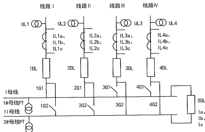
图 1 并列运行进线备自投方式
