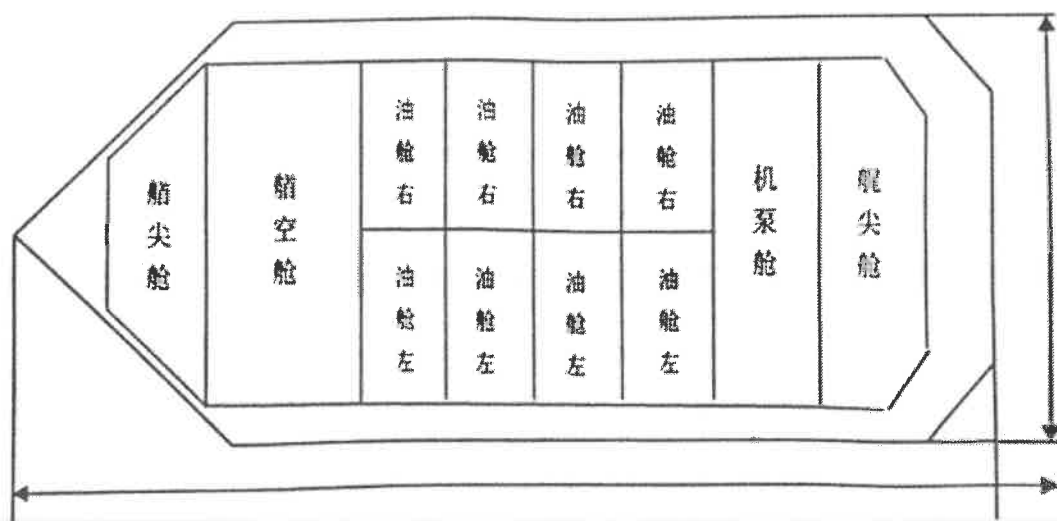
2.5-1金沙湾号船舱布局示意图
