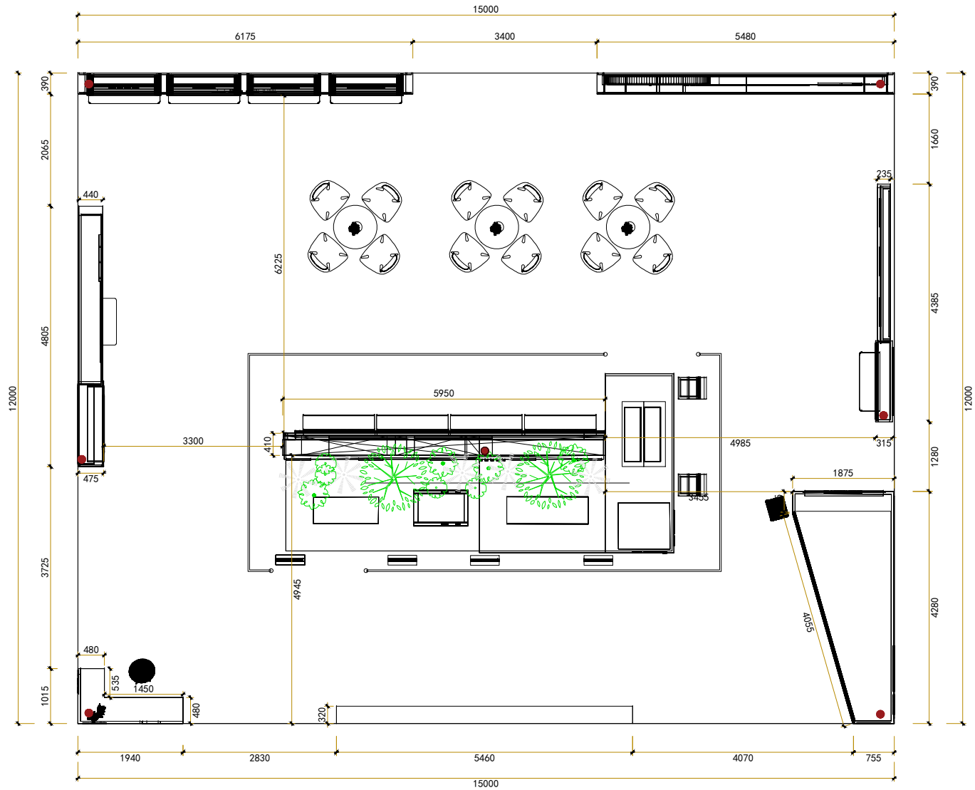
墙体尺寸放线图 1:60 面积约180平方 H=6000mm
