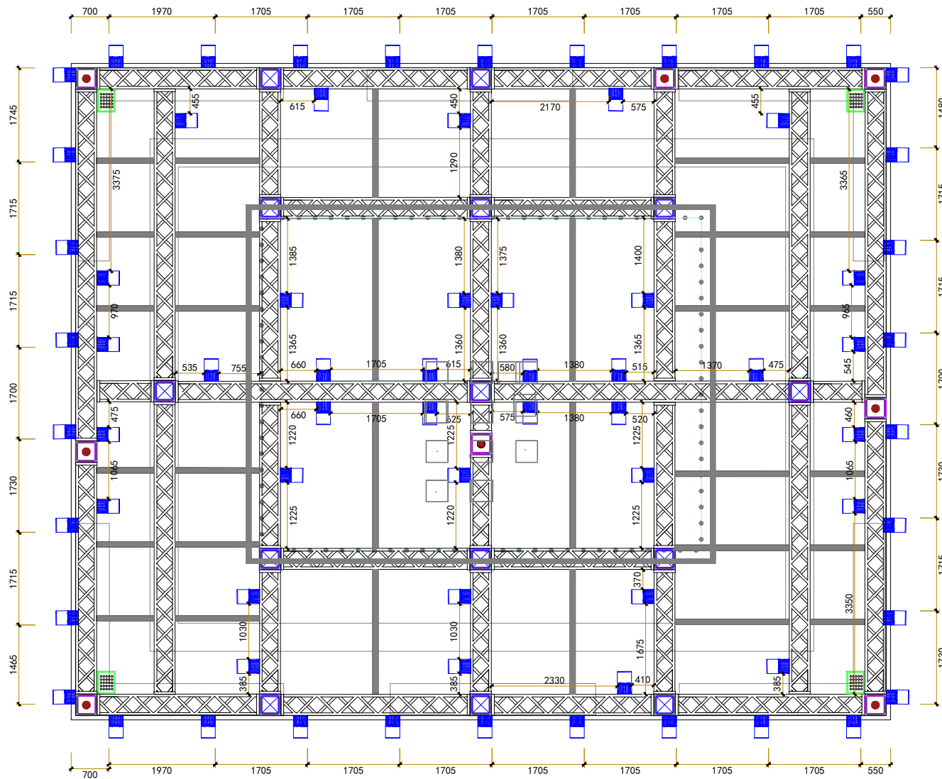
天花灯定位图 面积约180平方 H=6000mm
