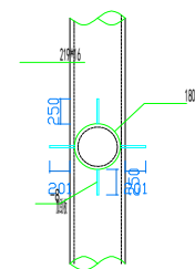
B-B 1:10
