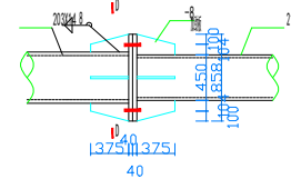
托架弦杆拼接节点示意 1:10
