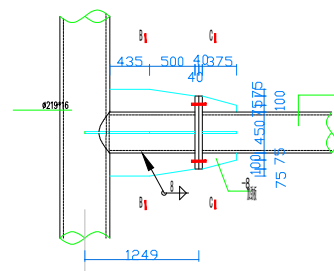
水平托架与钢柱连接节点示意 1:10
