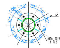
D-D 1:10
