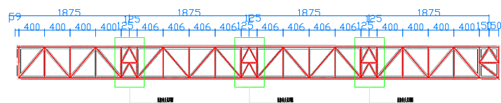
正视图 1:100
