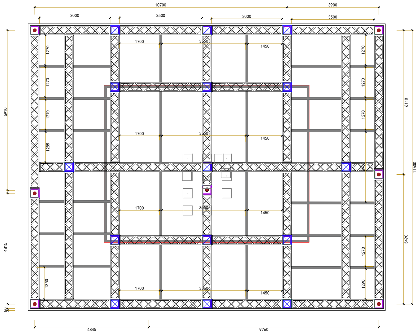
桁架结构落点图 1:60 面积约180平方 H=6000mm
